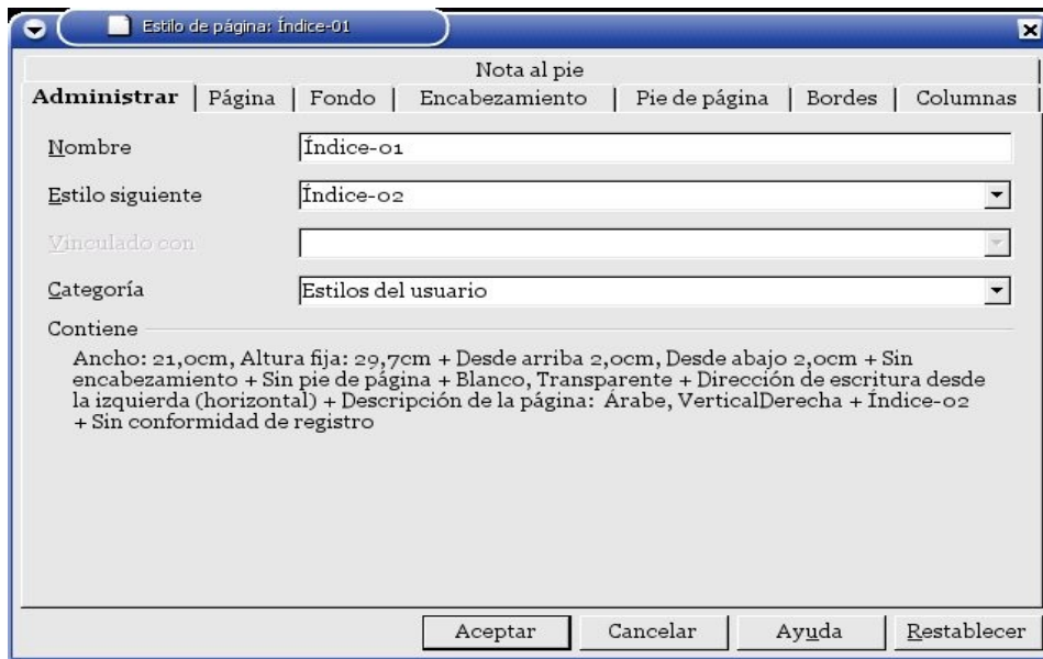
Figura 7: Pestaña «Administrar» para el estilo de página «Índice-01»
