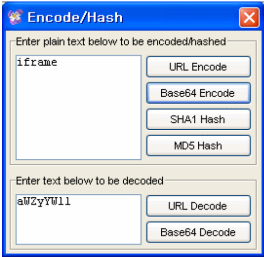
[ ] encode/hash
